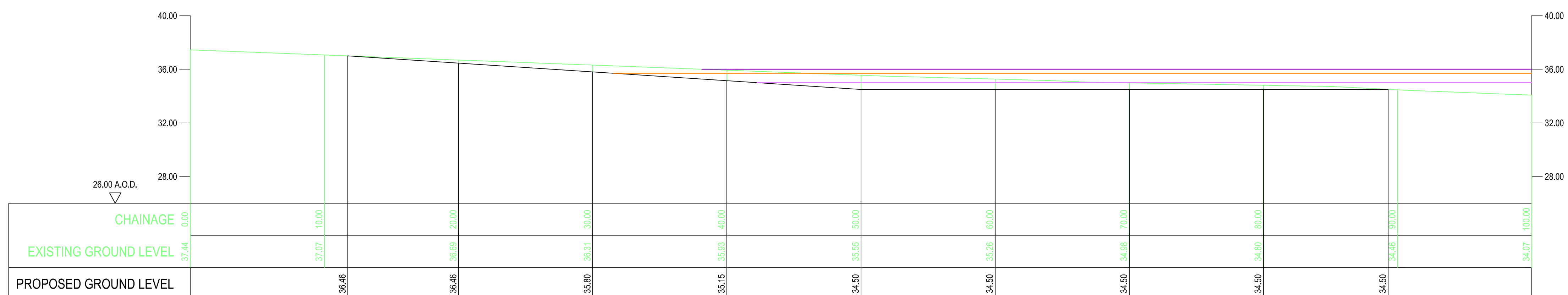
SECTION L HORIZ. 1:200 VERT. 1:200
